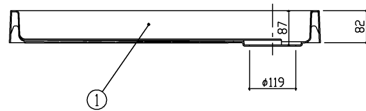
断面A-A
