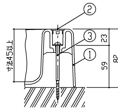
固定部詳細(1/3)
